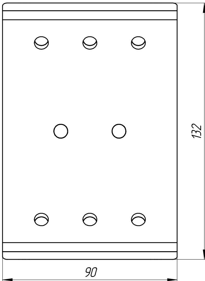
Колодка ТКГ-200
